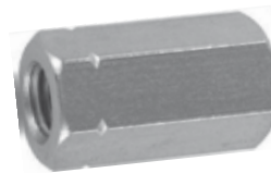
Hexagon coupling nut DIN6334 AISI 304
